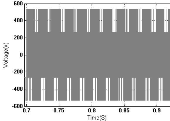
Fig. 8. STATCOM output voltage.
