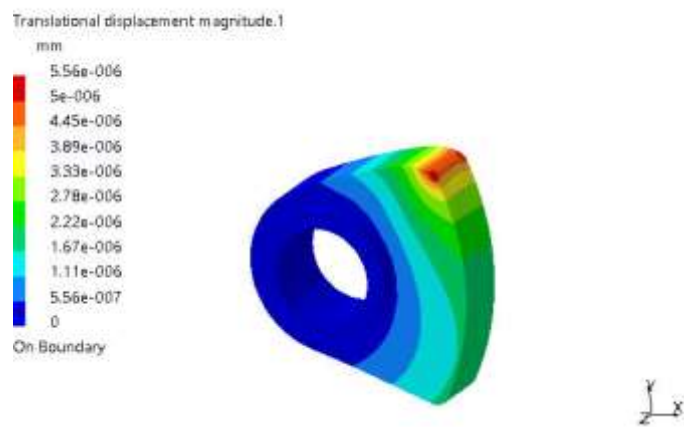
Fig. Crankshaft
