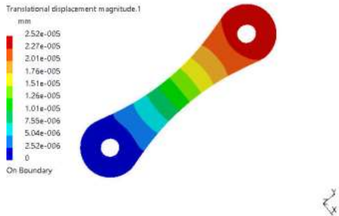
Fig. Connectingrod
