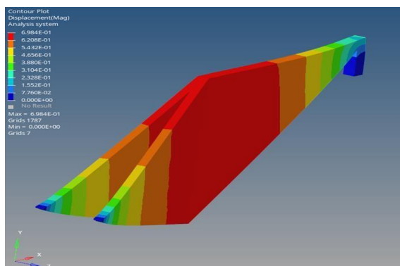
Fig. 16. Maximum displacement
