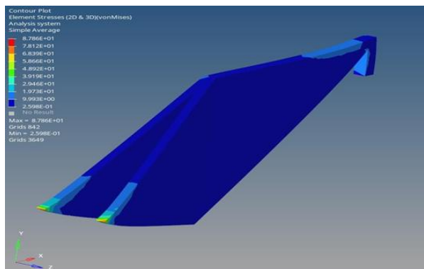
Fig. 17. Von mises stress
