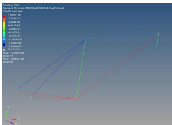
Fig. 15. Von mises stress of bamboo bike frame
