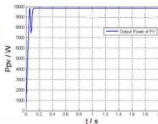
(d) Output power of PV array
