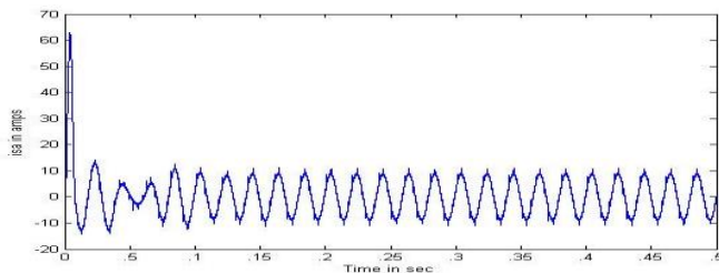
Fig. 8(d) Source current
