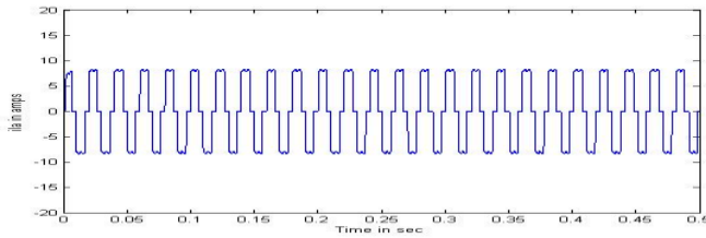
Fig. 8(b) Load current
